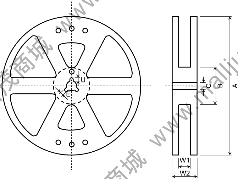
Fig. 16.3.6.1 Reel Dimensions
