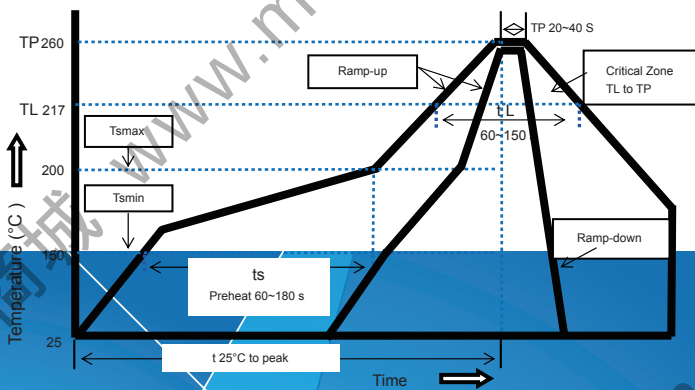
Soldering Parameters
