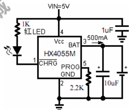
500mA 单节锂离子电池充电器
