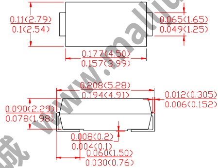
SMA(DO-214AC)
