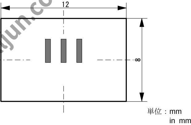
第2図 たわみ試験用基板 Figure 2. Test Board for Bending Strength Test
